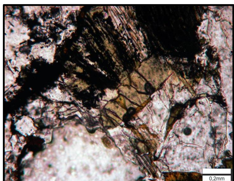
Cristal de turmalina perpendicular à xistosidade. Nicóis paralelos.
