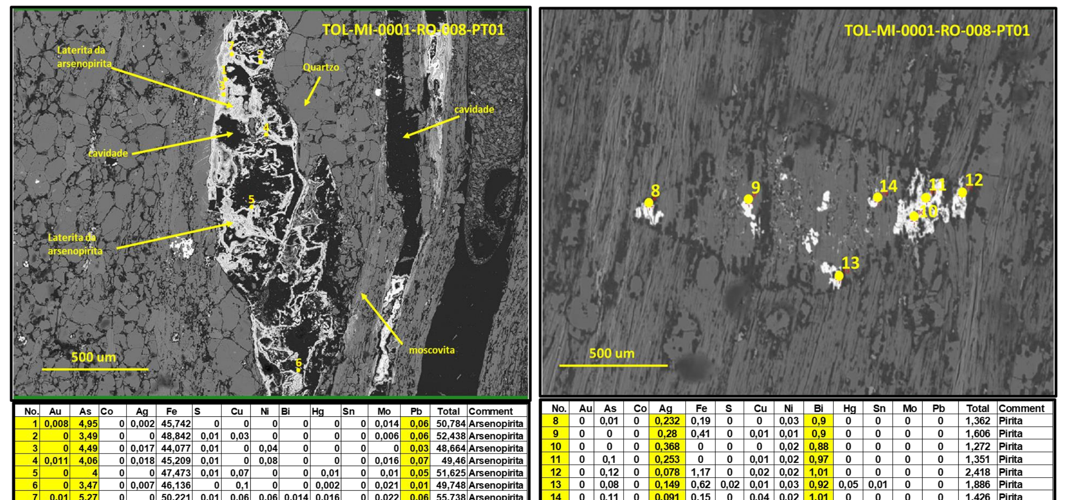
Imagem e o resultado analítico da microsondagem nos porfiroblastos de arsenopirita e pirita. A identificação do Ouro, anomalia de Ferro, anomalia de Arsênio, Prata e Bismuto juntos. (Microsonda Eletrônica JEOL JXA-8230, 5 WDS e 1 EDS/DEGEO/EM/UFOP).
