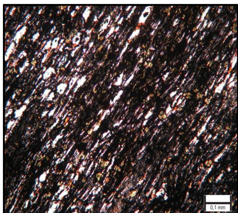
Texturas lepidoblástica e nematoblástica. Nicóis cruzados.
