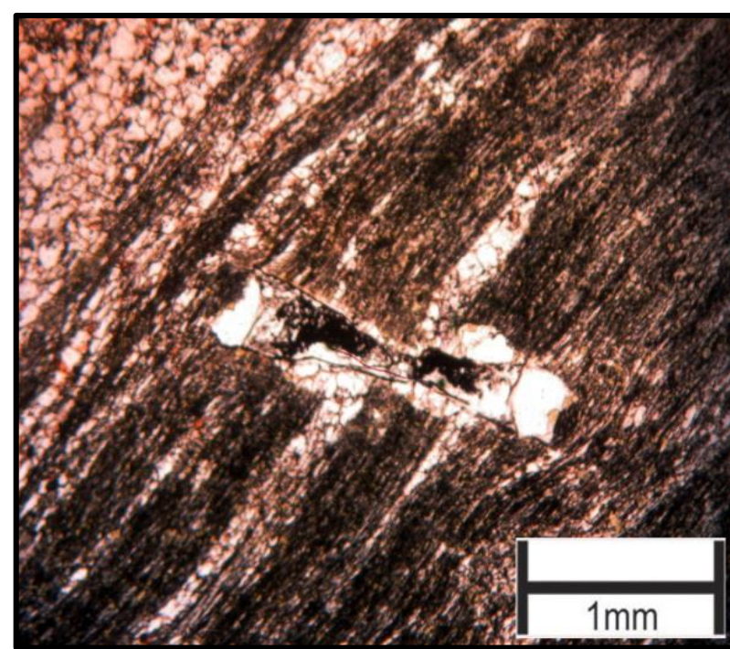
Porfiroblasto de arsenopirita, alterados perpendicular à xistosidade. Nicóis paralelos.
