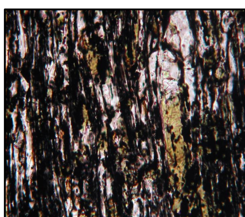
Cristais de turmalina e quartzo estirados segundo a xistosidade. Nicóis paralelos.
